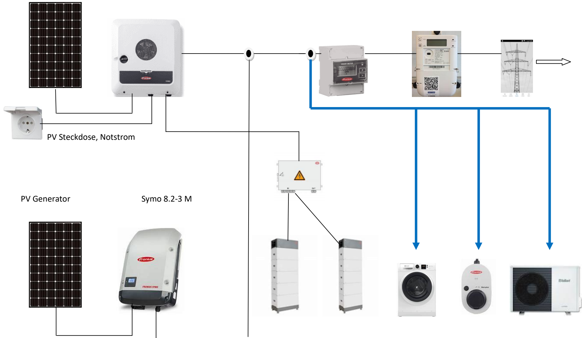
SYMO GEN 24/8
